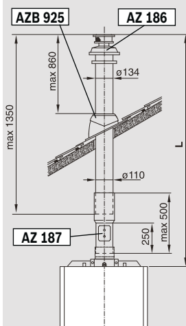
Svislé provedení bez kolen, šikmá střecha
