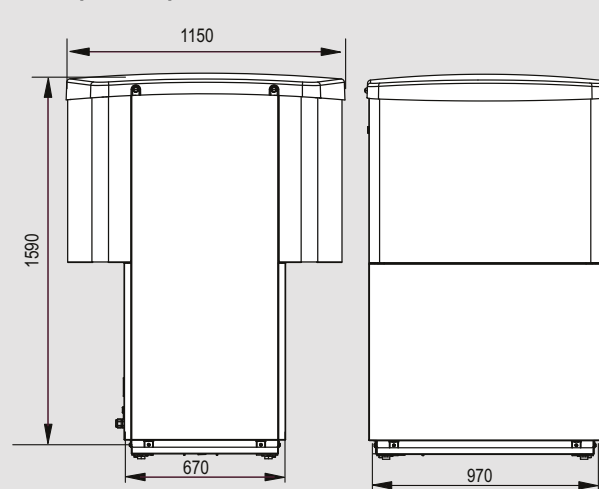
Teplné čerpadlo SAO ...-1
