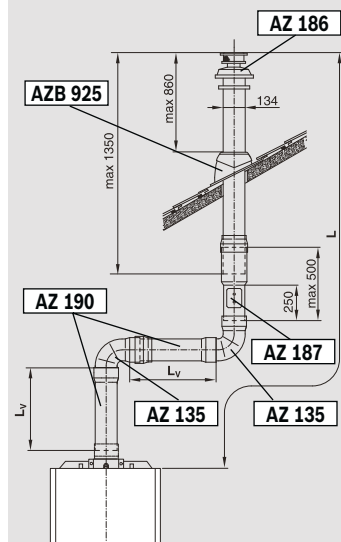
Svislé proved. s koleny 2x 90°, šikmá střecha
