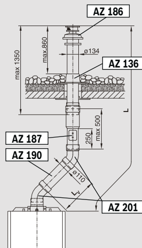
Svislé provedení s koleny 2x 45°, vodorovná střecha
