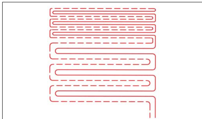
Obr. 3-9 Forma pokládky dvojité meandr s integrovanou zhuštěnou okrajovou zónou
