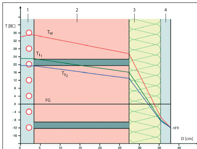
Obr. 4-25 Porovnání průběhů teplot ve vícevrstvé vnější stěně s hodnotou U < 0,35\text{ W/m}^2\text{K}
