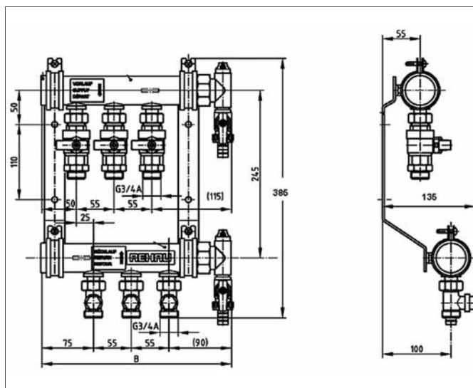
Obr. 9-36 Rozměry
