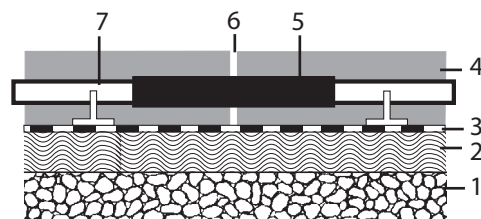
Správné vedení topné trubky UNIVERSA v místě dilatační spáry
