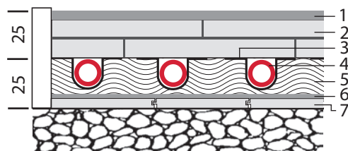
Skladba konstrukce se suchou podlahou
