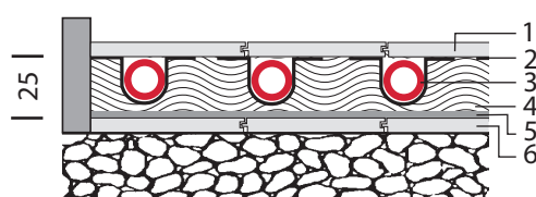
Skladba konstrukce s dřevěnou podlahou
